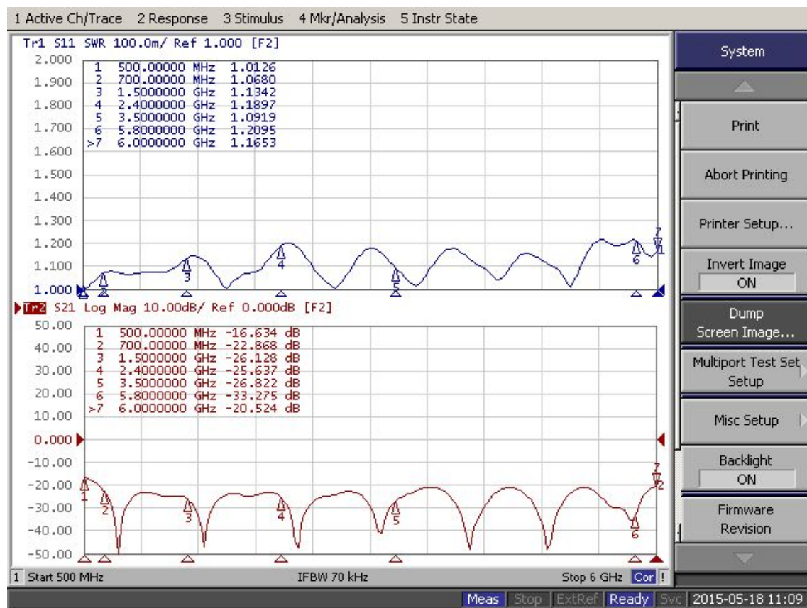
b) 输出驻波及隔离度
