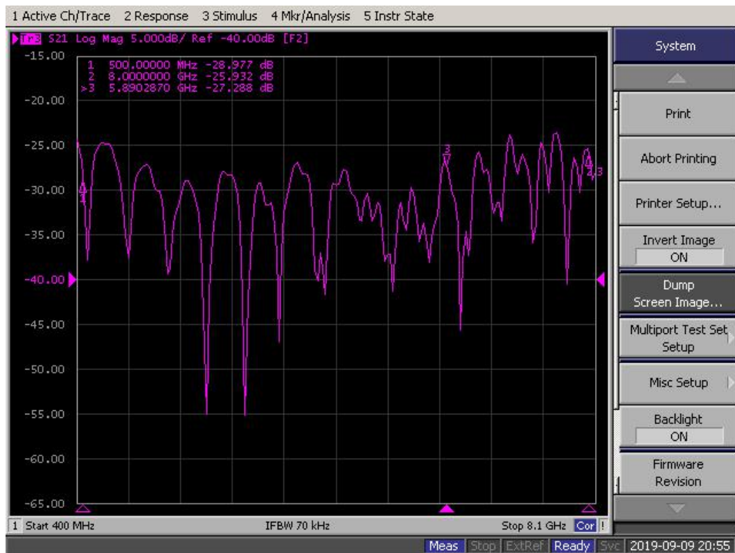
一分八功分器测试截图（隔离度）
